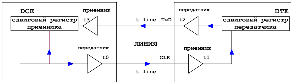
Рис. 27. Путь прохождения синхронизации и данных
