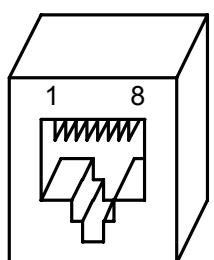
RJ-45 Розетка
