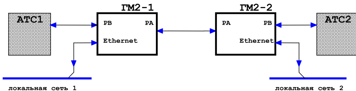
Рис. 26 Вариант построения сети передачи данных на основе мультиплексов ГМ
