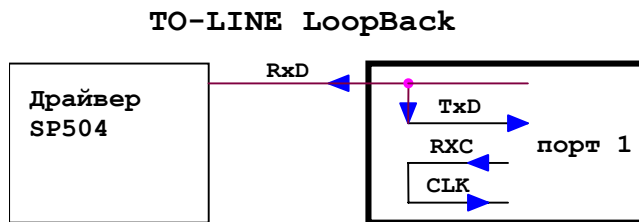
Рис. 45. Структура шлейфа TO-LINE для порта 1
