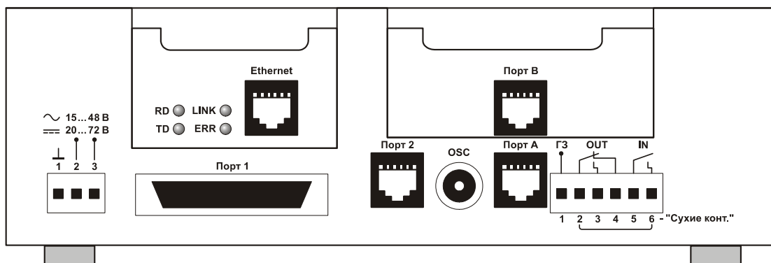
Рис. 5. Вид задней панели мультиплексора ГМ с установленными модулями Ethernet и порта В (второй Е1)
