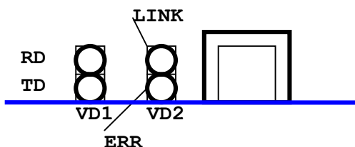
Рис. 6. Положение светодиодов на модуле ГМ-2-МБЕ (одноканальный вариант модуля)
