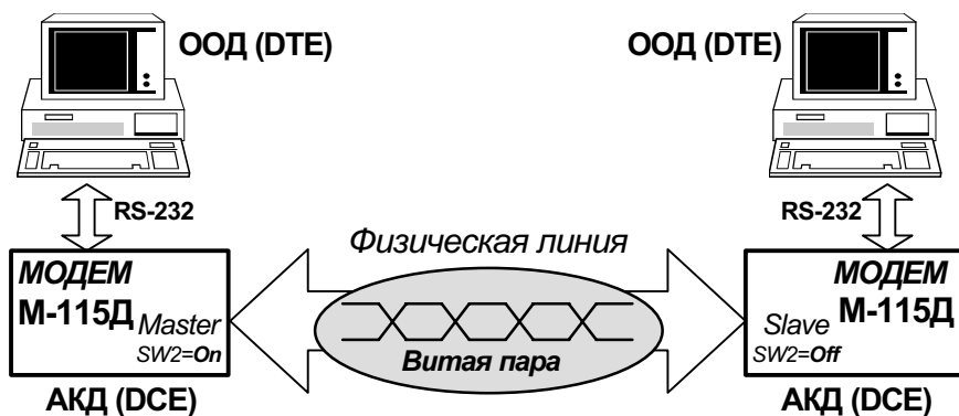
Рис. 1. Организация канала связи с помощью модемов М-115Д
