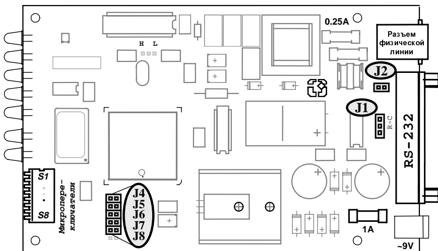
Рис. 3 Расположение элементов на плате модема
