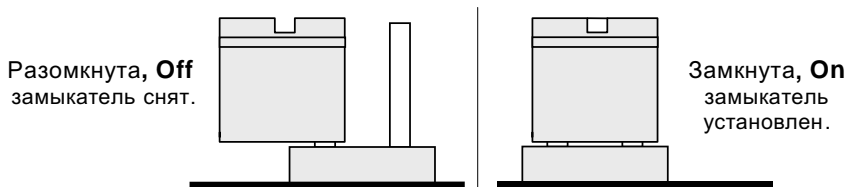
Рис. 7 Положение замыкателя на перемычках J2, J4...J8
