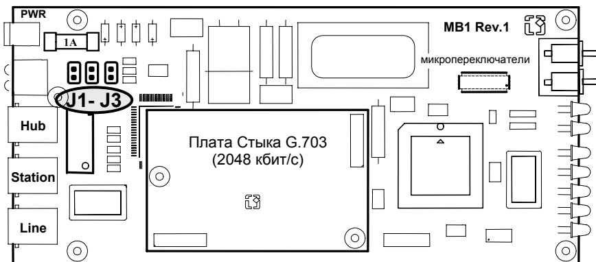
Рис. 7 Расположение элементов на плате модема
