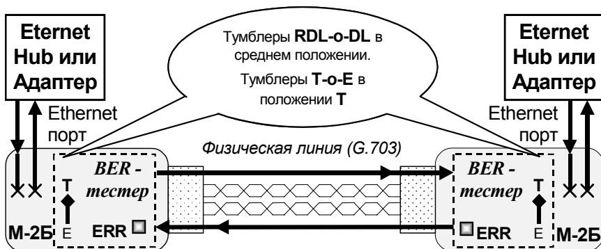
Рис. 11 Применение BER–тестера
