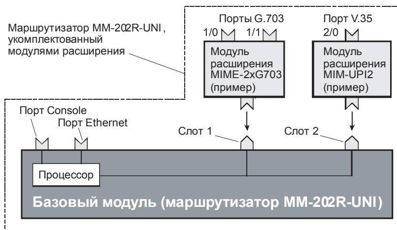
Рис. 1. Структура маршрутизатора MM-202R-UNI и подключение к нему модулей расширения
