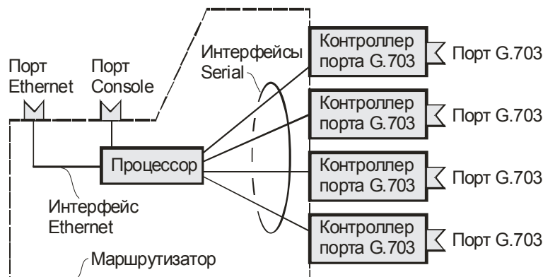
Рис. 2. Внутренние интерфейсы маршрутизатора и контроллеры портов
