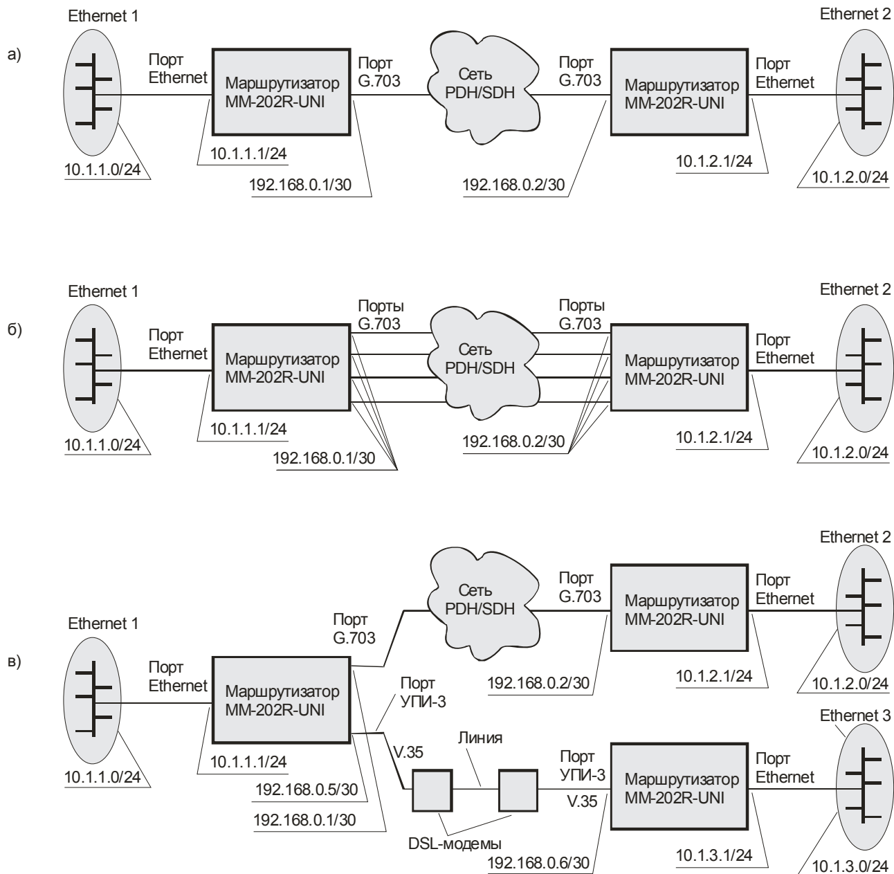
Рис. 3. Примеры построения систем с использованием маршрутизатора MM-202R-UNI
