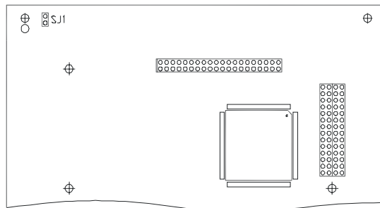
Рис. 4. Расположение переключателя SJ1 на основной плате маршрутизатора настольного исполнения
