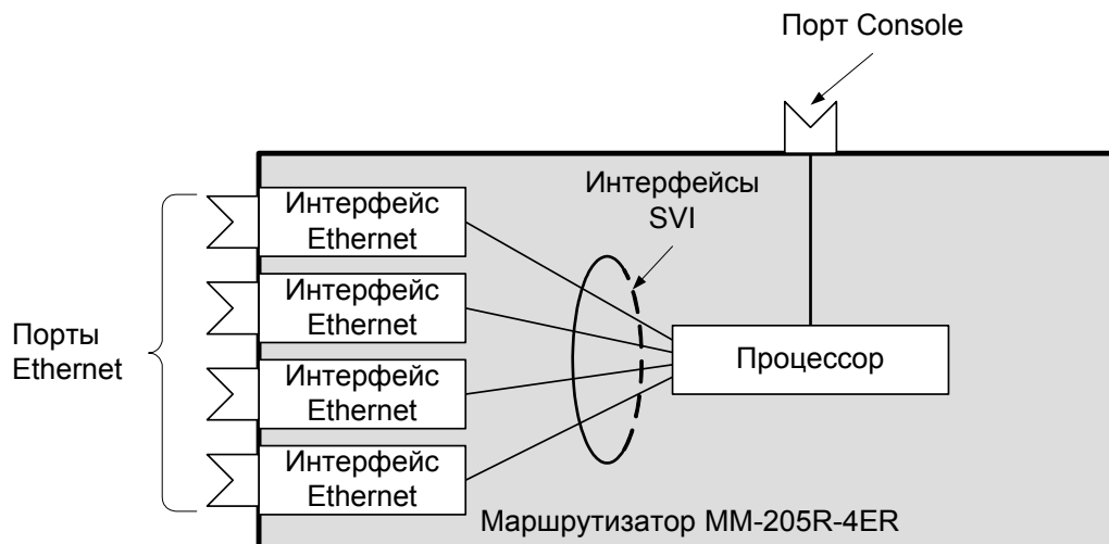
Рис. 2. Внутренние интерфейсы маршрутизатора
