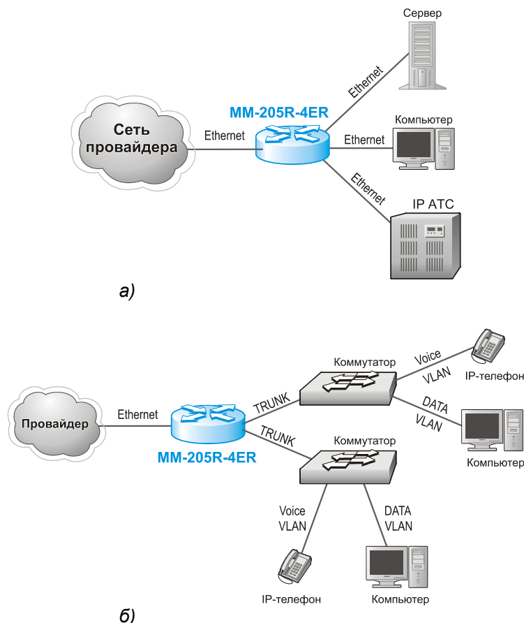
Рис. 3 Примеры построения сетей с использованием маршрутизатора MM-205R-4ER
