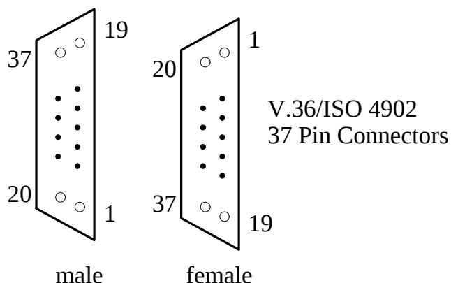
37-контактные разъемы V.36/ISO 4902
