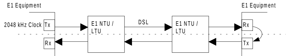
Рисунок 4-2: Синхронная работа (= "синхронизация по шлейфу).
