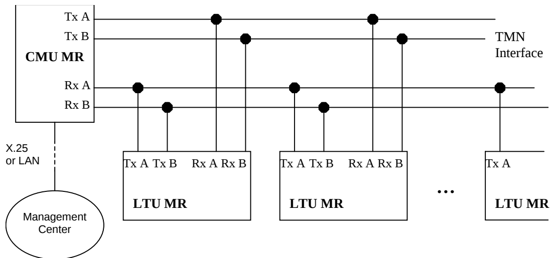
Рисунок 4-9: 4-проводное соединение шины TMN для устройств типа Minirack.
