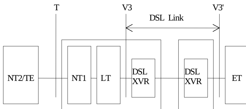
Рисунок 4-4: Опорные точки PRA.
