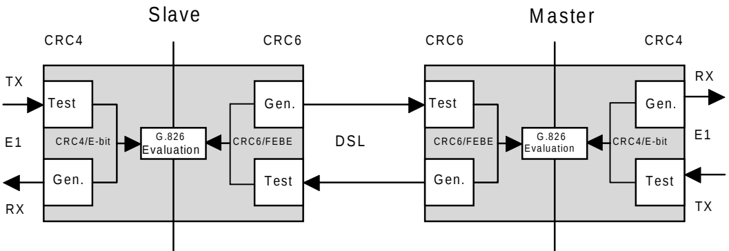
Рисунок 5-13: Оценка параметров E1 в соответствии с G.826.
