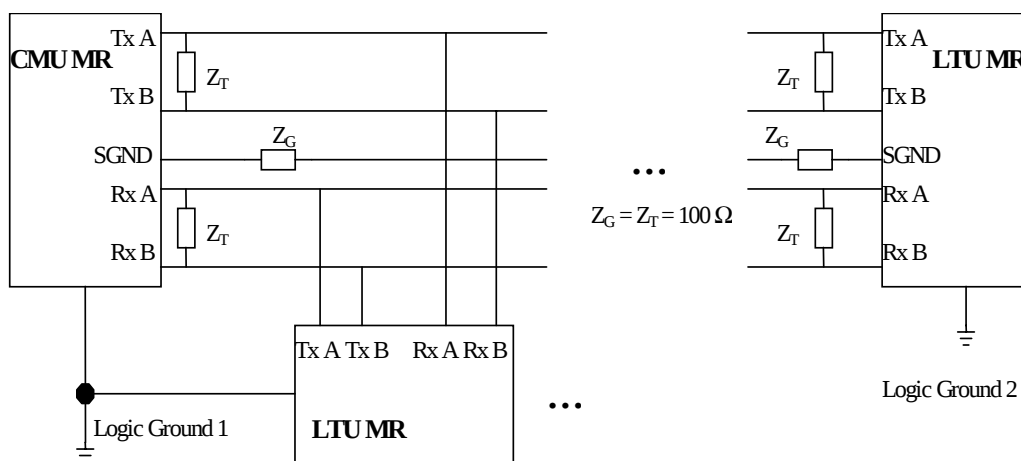
Рисунок 4-12: Согласованная нагрузка для протяженной шины TMN.
