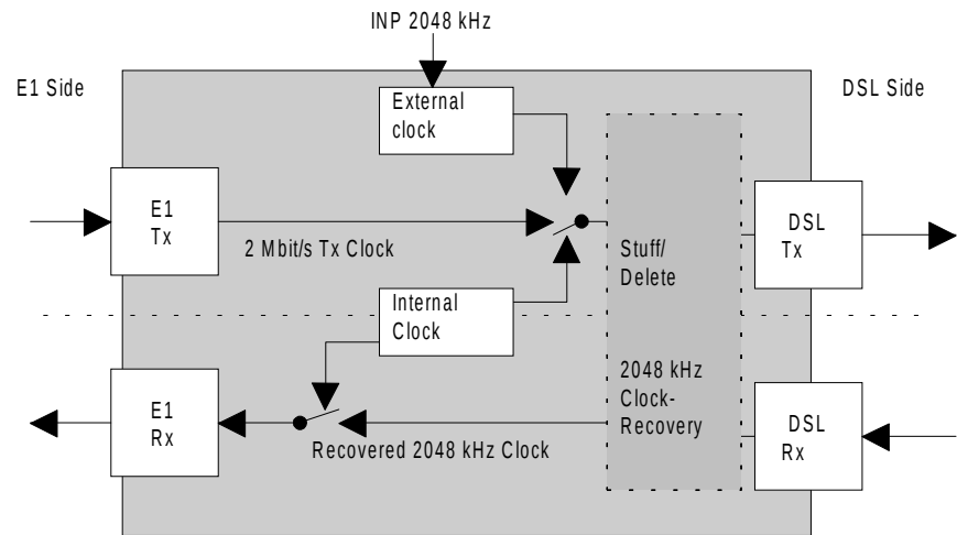
Рисунок 4-1: Источники тактовой частоты.
