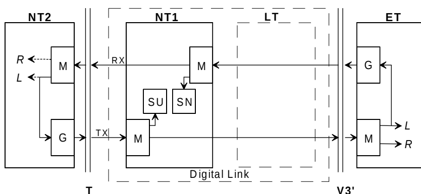
Рисунок 4-8: Цифровая линия передачи данных с текущим контролем CRC в NT1
