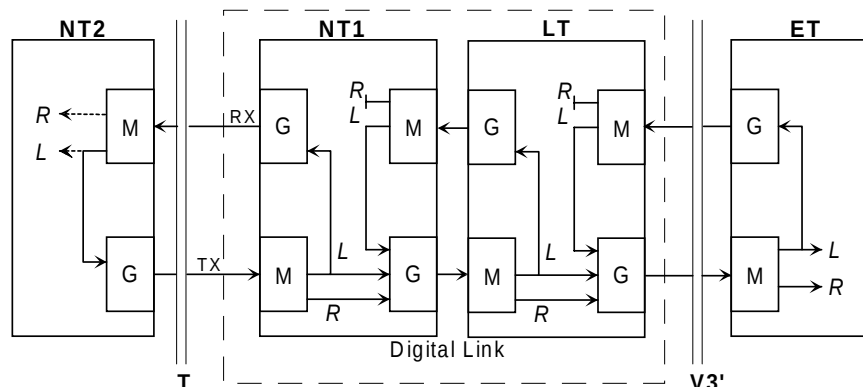
Рисунок 4-7: Цифровая линия передачи данных с функцией CRC в LT и NT1.
