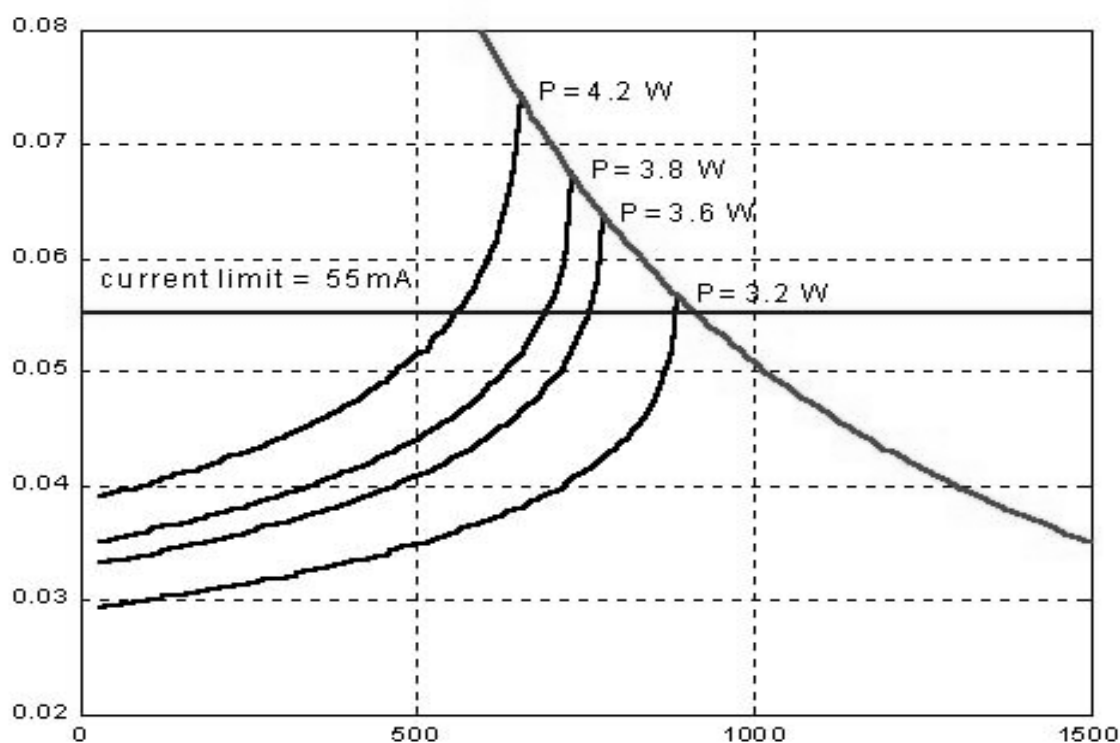
Рисунок 7-15: Зависимость тока линейного питания от сопротивления шлейфа для модулей NTU, потребляющих различную мощность.
