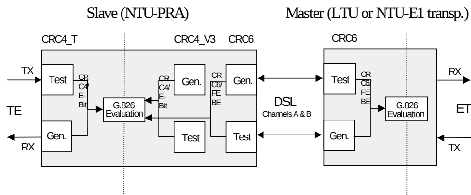
Рисунок 5-14: Оценка параметров PRA в соответствии с G.826.
