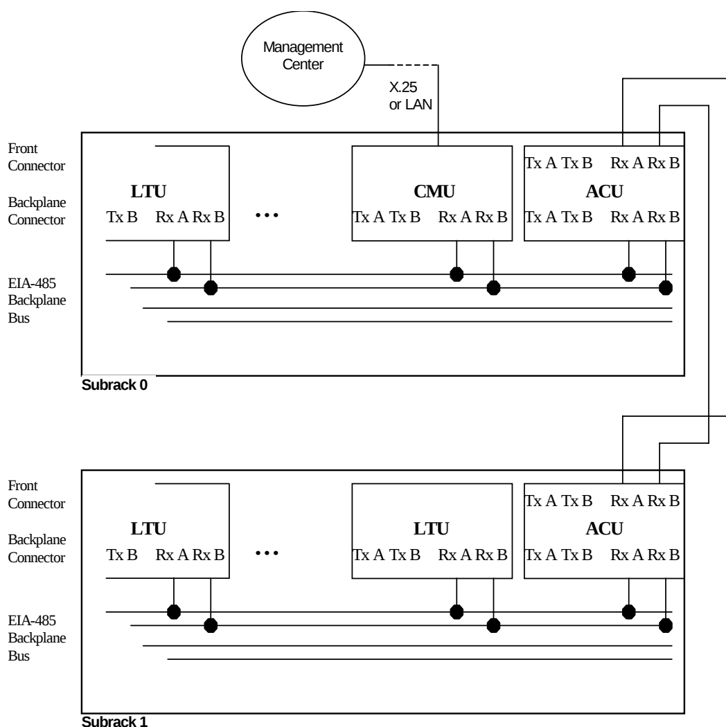
Рисунок 4-11: 2-проводное соединение шины TMN для съемных модулей, устанавливаемых в модульную кассету.
