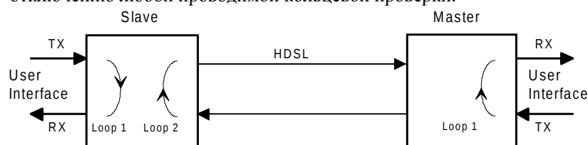
Рисунок 13-19: Стандартные проверки по шлейфу.
