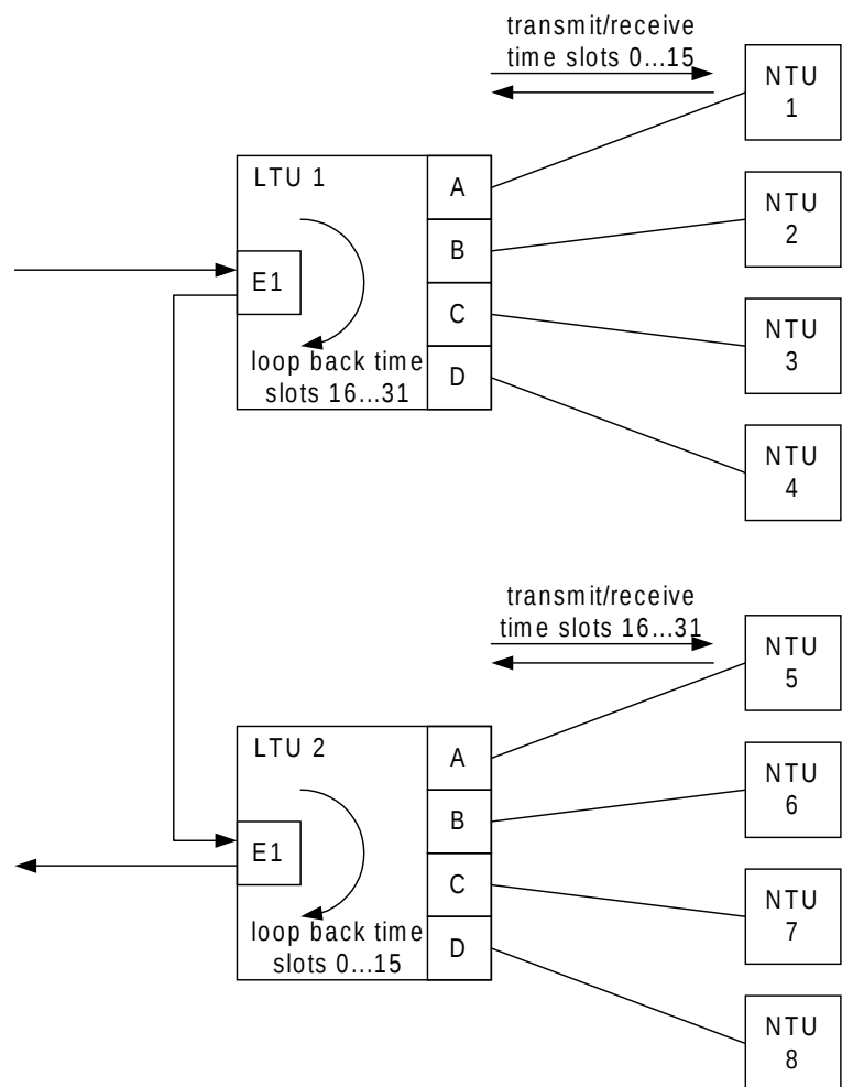
Рисунок 9-18: Каскадное подключение модулей Multipoint LTU.
